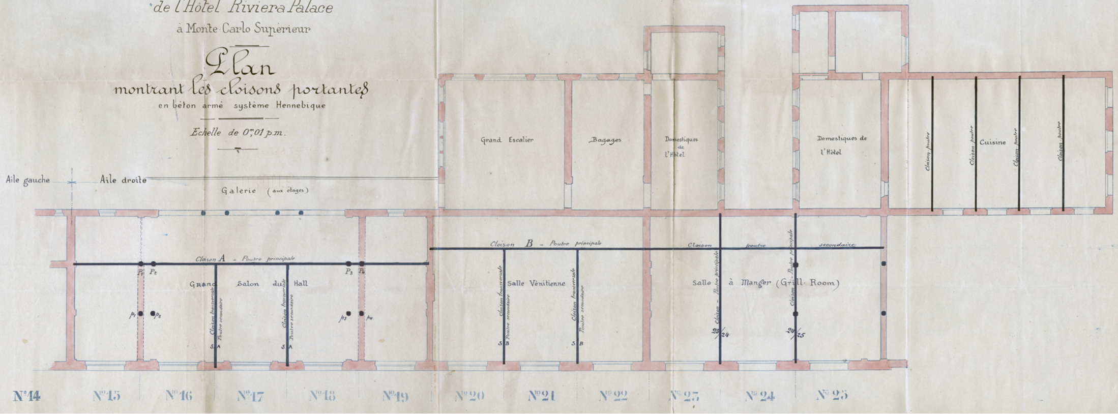
13.12 Plan de réalisation en béton armé de l'Hôtel Riviera Palace, AD06 3U1 1193
