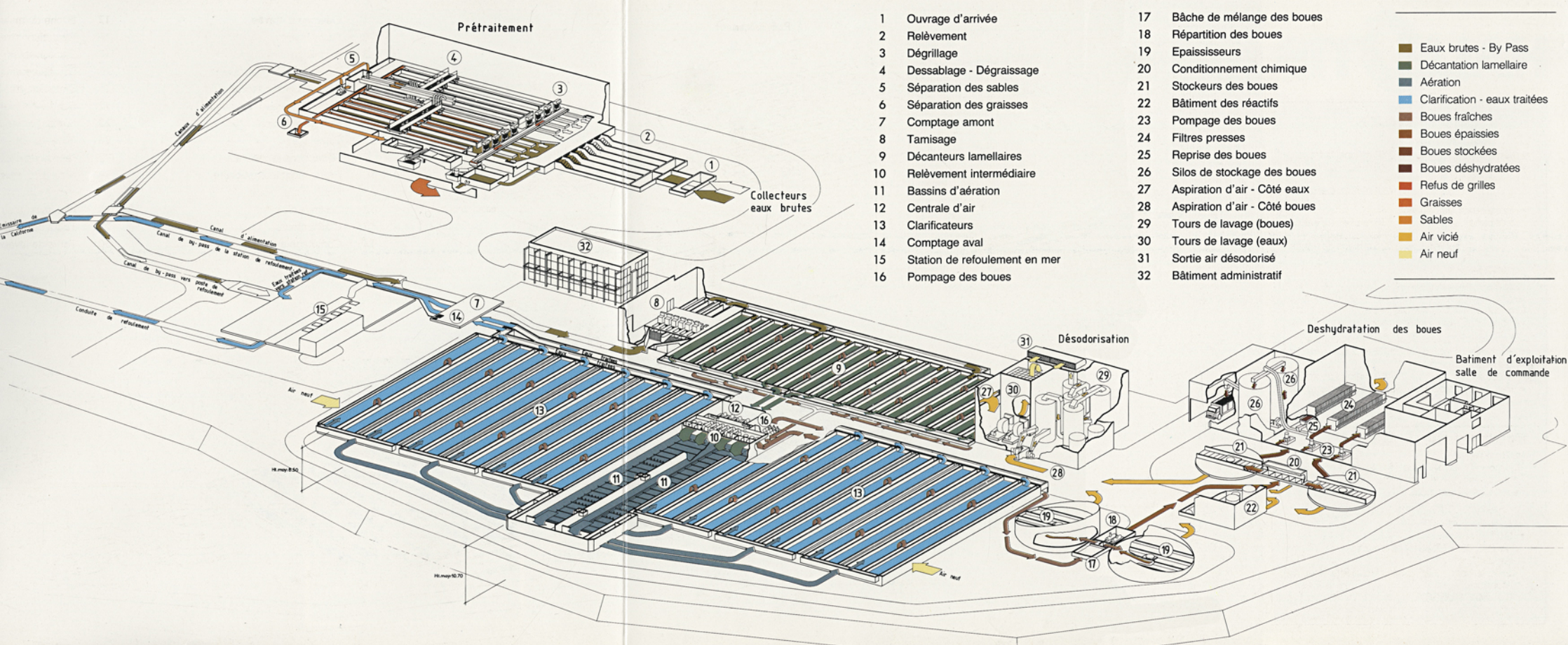
10.6 Schéma de fonctionnement de la station d'épuration des eaux usées de la ville de Nice Haliotis, s.d., vers 1990
