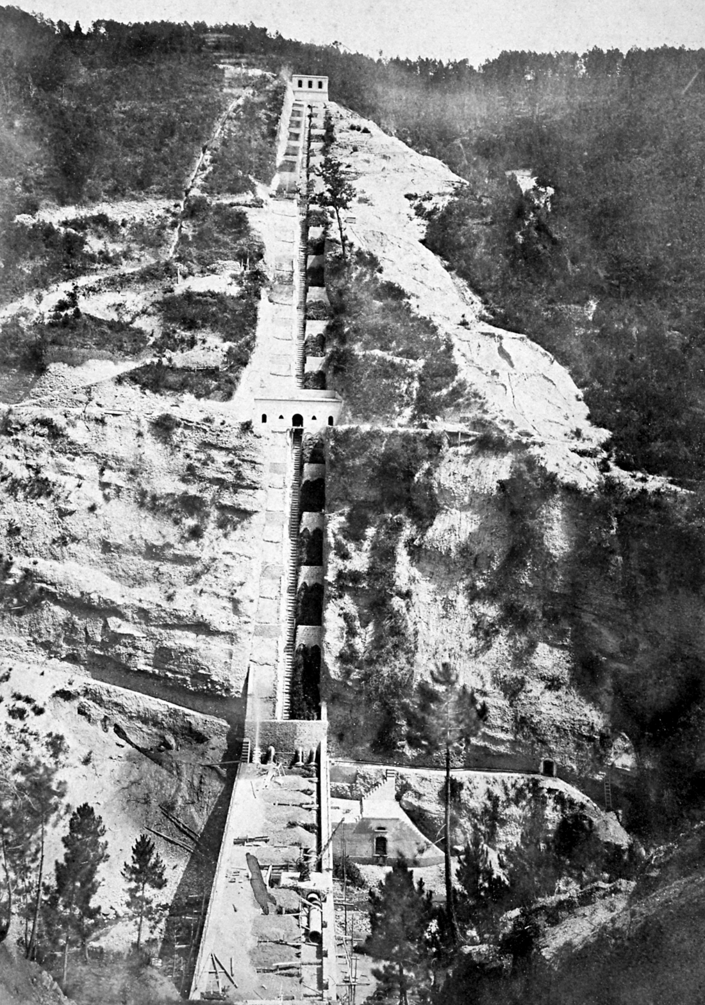
5.6 Construction du canal de la Vésubie, vers 1880. © Bibliothèque de Cessole
