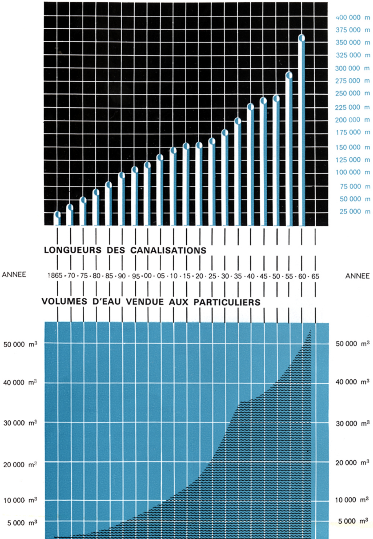
6.2 Courbe d'évolution de la consommation d'eau et d'extension du réseau de canalisation d'eau potable à Nice de 1865 à 1960
