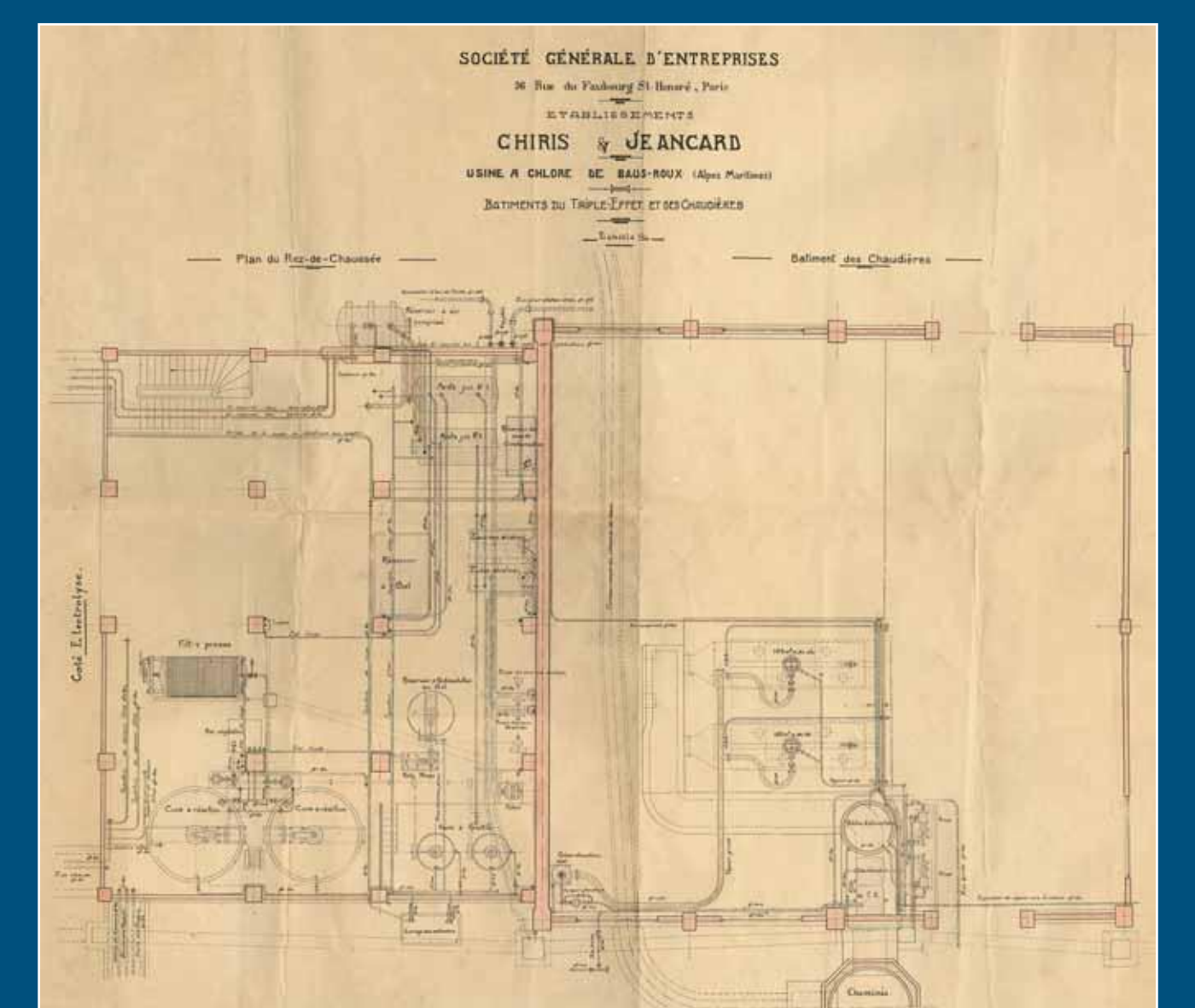
Plan de l'usine de chlore de l'entreprise Chiris à Baus Roux, 1917. AD06. 32 J 155.
